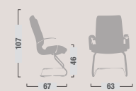
Z 78 Poltrona attesa fissa con braccioli. Fixed armchair.
